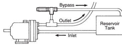
Fig. 1: Off-Line
