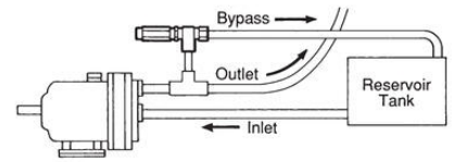
Fig. 1: Off-Line
