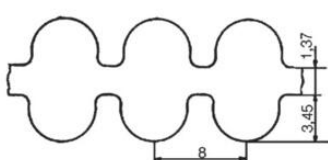
Kuggrem HTD D8M
