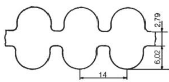
Kuggrem HTD D14M
