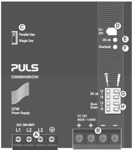
Fig. 15-1 Front side
