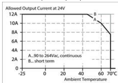
Kuormitettavuus (virta/lämpötila)
