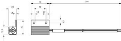
Thermostat KTO 011 (NC)
