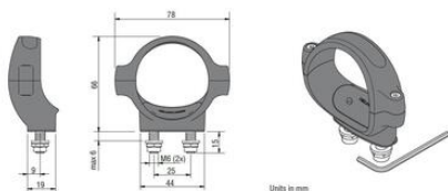
Dimensions
