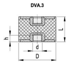
DVA.3 - 8 - 8 - M3 - 55 D L d Shore A
