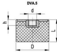
DVA.5 - 10 - 10 - M4 - 55 D L d Shore A
