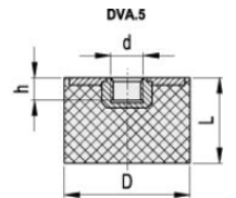
DVA.5 - 10 - 10 - M4 - 55 D L d Shore A
