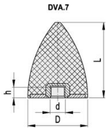
DVA.7 - 20 - 24 - M6 - 55 D L d Shore A
