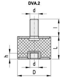
DVA.2 - 8 - 8 - M3 - 6 - 55 D L d Shore A
