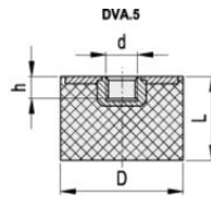
DVA.5 - 10 - 10 - M4 - 55 D L d Shore A
