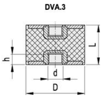
DVA.3 - 8 - 8 - M3 - 55 D L d Shore A
