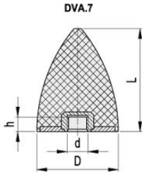
DVA.7 - 20 - 24 - M6 - 55 D L d Shore A
