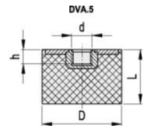
DVA.5 - 10 - 10 - M4 - 55 D L d Shore A
