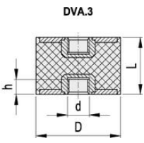
DVA.3 - 8 - 8 - M3 - 55 D L d Shore A
