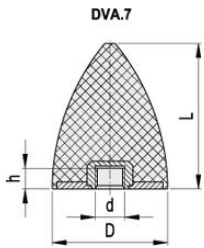
DVA.7 - 20 - 24 - M6 - 55 D L d Shore A
