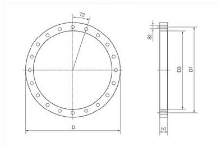
iglidur® PRT spacer ring_POM
