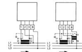
PQ33/PL33
