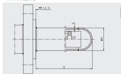
■ Thermowell (option)
