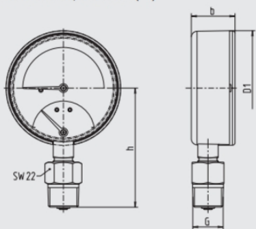
Model 100.01.80, lower mount (LM)
