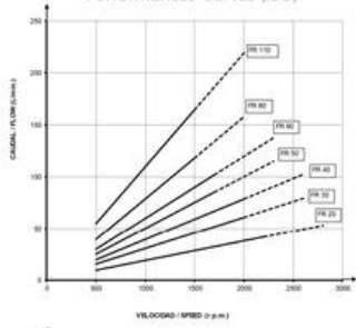
Curvas de Rendimiento (ISO) Performances Curves (ISO)
