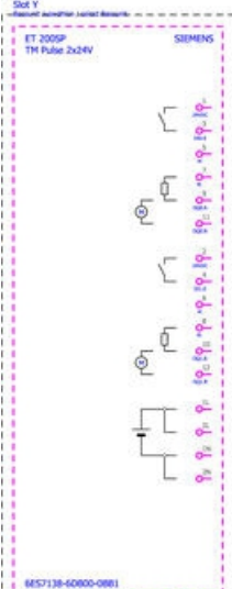
ET 200SP TM Pulse 2x24V
