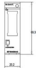
Oben / Top
