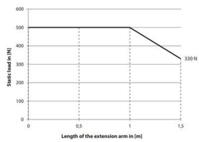
Load diagram for static load capacity CS-480 B.fle
