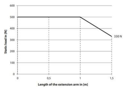
Load diagram for static load capacity CS-480 B.fle
