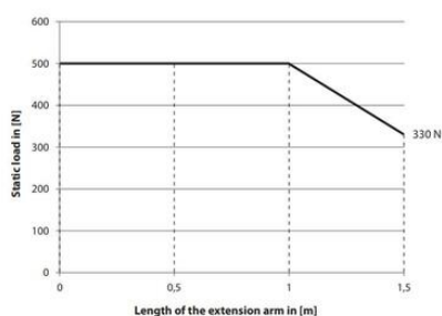
Load diagram for static load capacity CS-480 B.fle X
