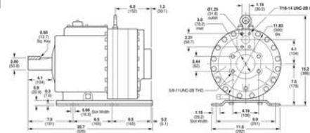
D-35 Models with SAE Flange Intert/Outlet Por
