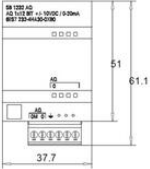
Vorne / Front
