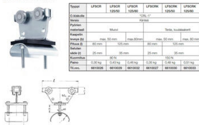
Metallinen lattakaapelivaunu
