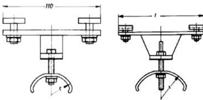
Technische Daten der Endtragen „FECR“ und „FECRS“ Technical data sheet of the end supports "FECR" and "FECRS"
